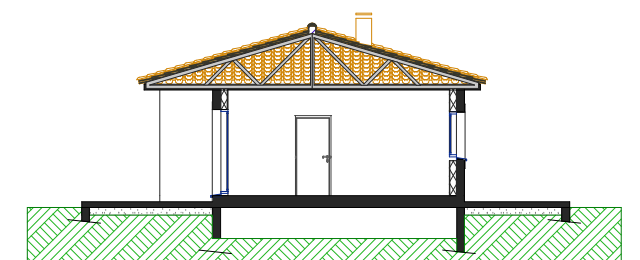
Coupe type
