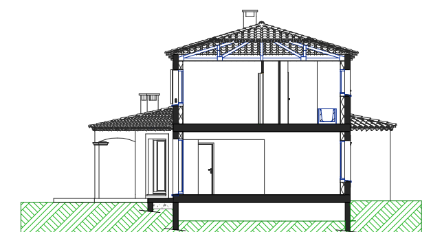
Coupe type
