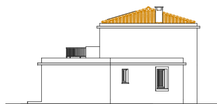
ELEVATION EST
