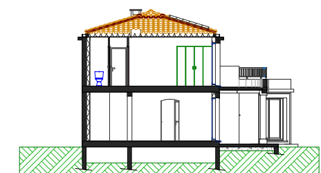
Coupe type
